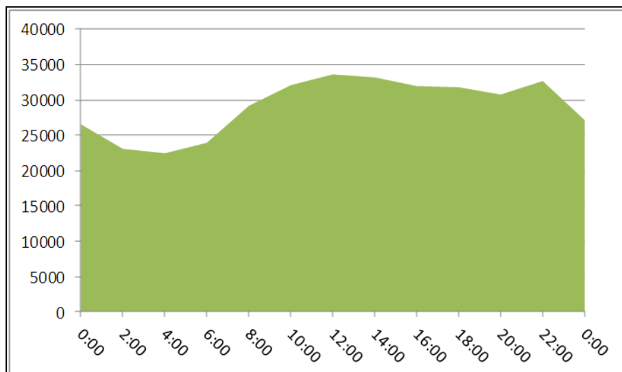
Figura 3. Curva prevista de demanda de energía eléctrica (MW/h). 11 de mayo de 2011 (Fuente: REE).
